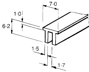
P.C.B. Handle/Board Stiffener, Aluminium.
